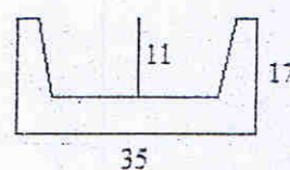
Korytko długie 70 x 35 x 17/ 11 cm
