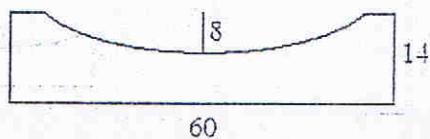
Płytkościek 60 x 50 x 14/ 8 cm
