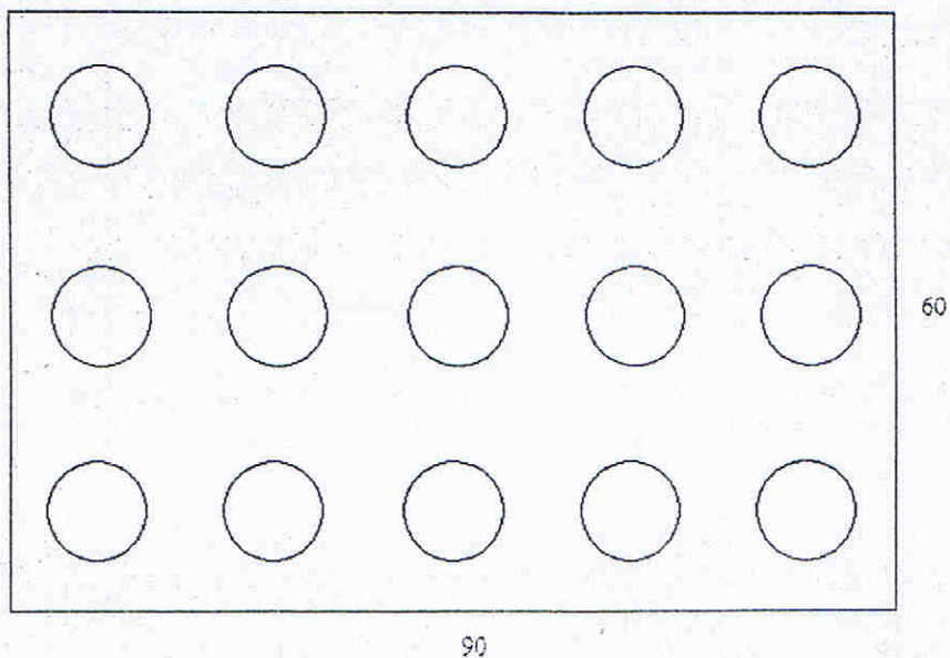
Płytki ażurowe 90 x 60 x 10 80 x 50 x 10
