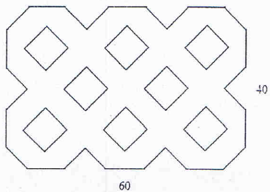
Płytki ażurowe 60 x 40 x 8 60 x 40 x 10
